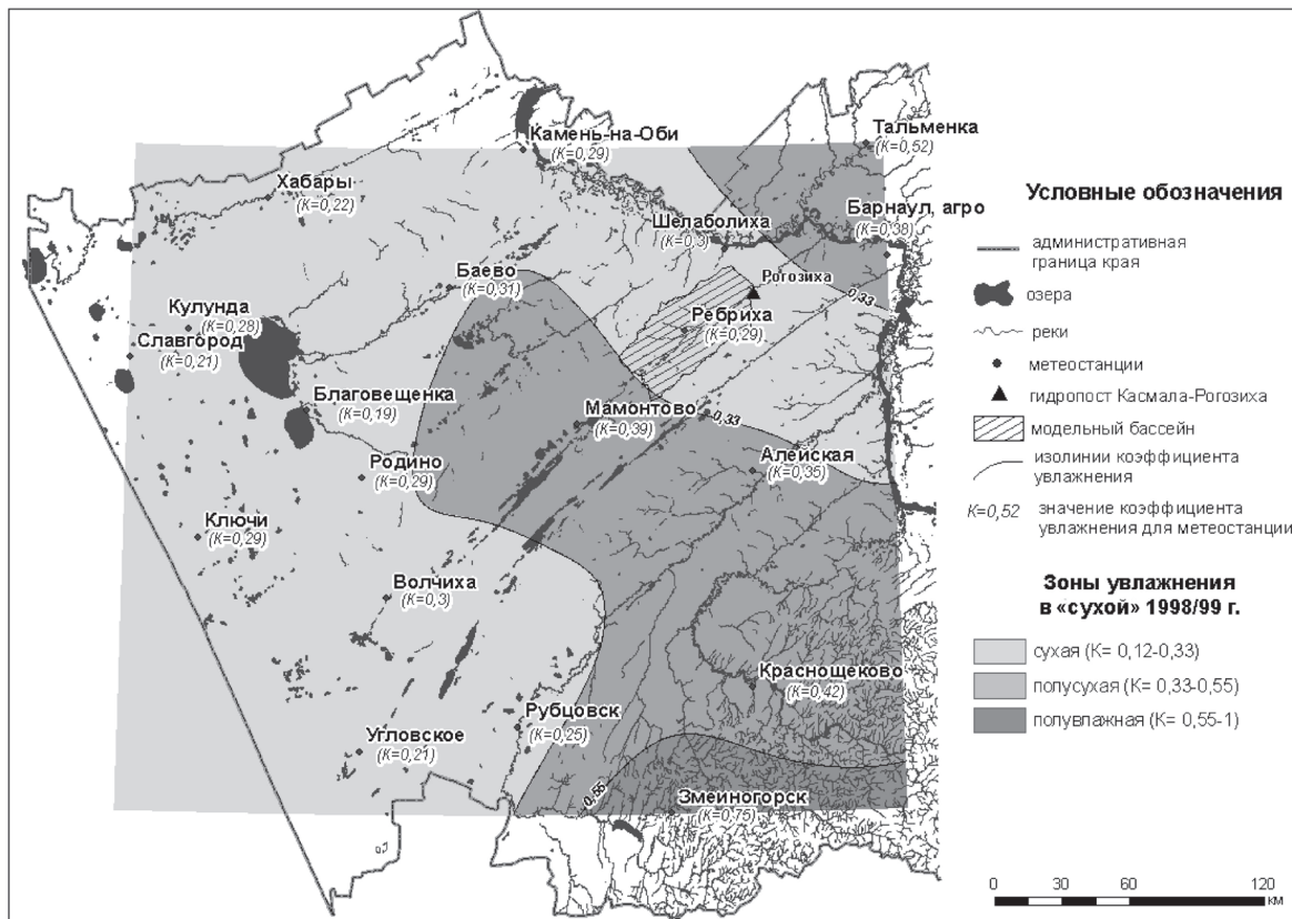
Рис. 6. Распределение атмосферного увлажнения в «сухой» период – 1998/99 г.
